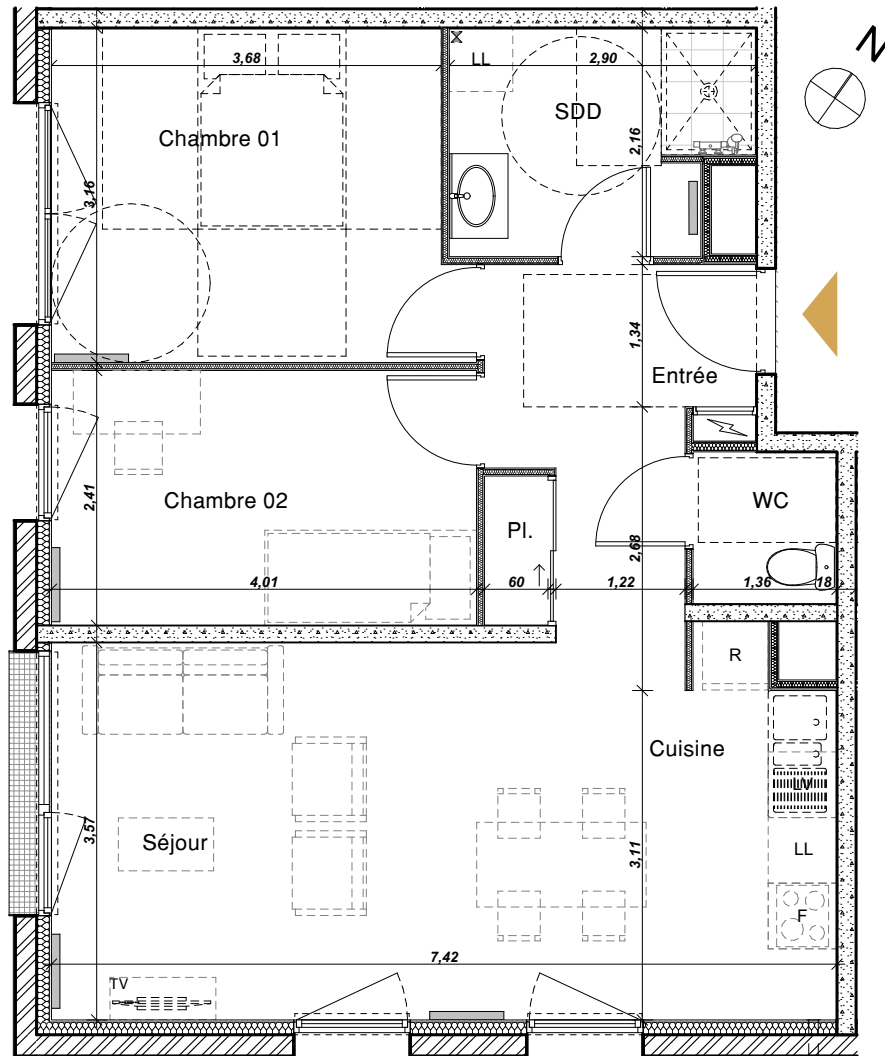
Plan de niveau - RDC
