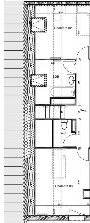
Plan de niveau - R+2 et R+2+Combles
