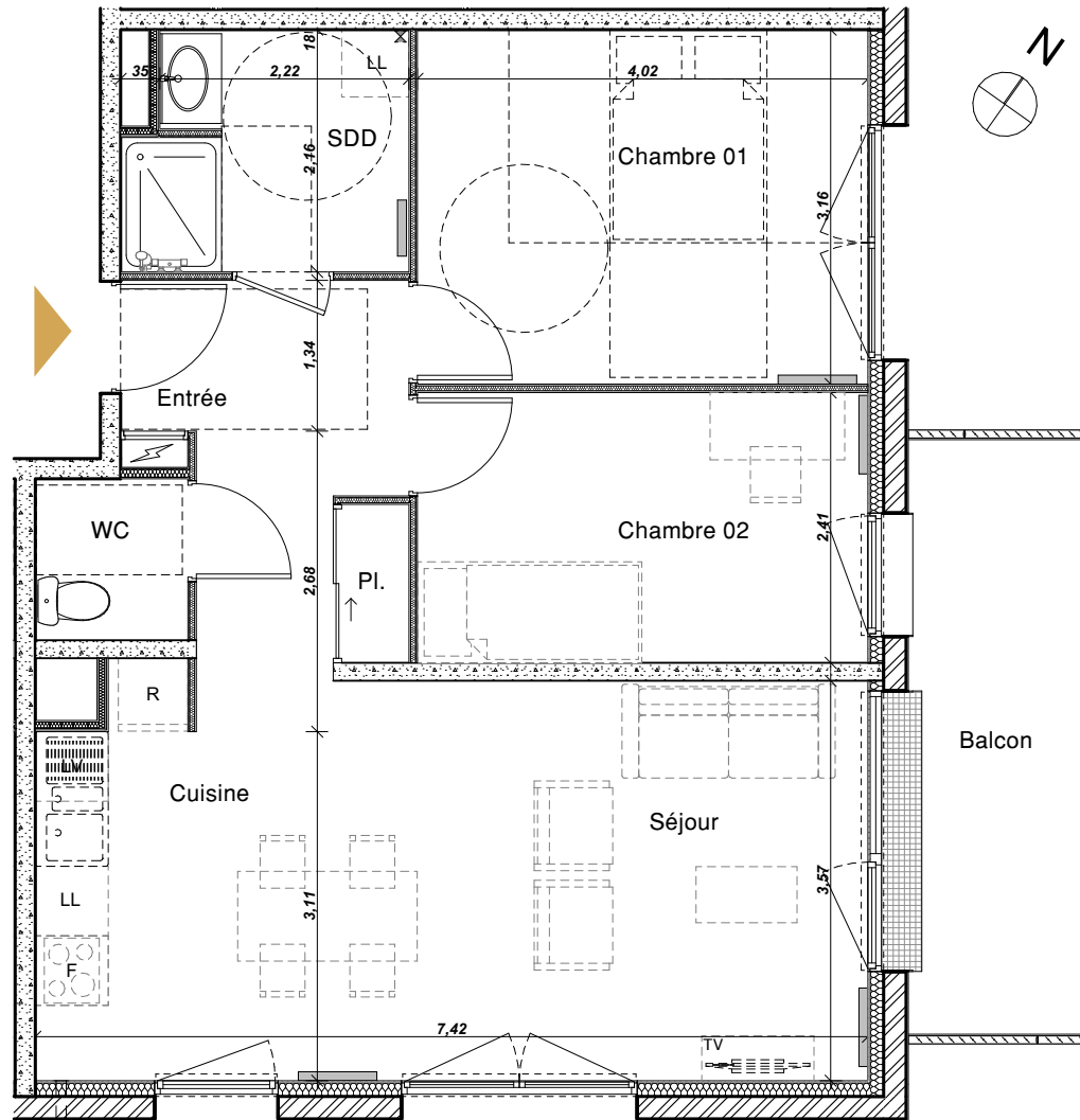
Plan de niveau - R+1
