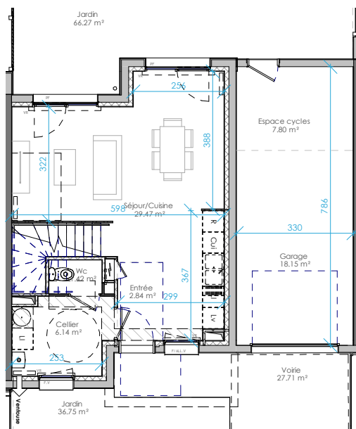
NORD 1 : 150
